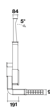
Vista laterale installazione con motore Slim posteriore
