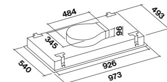
Motore sottotetto installato sulla cappa
