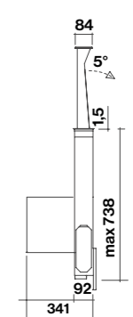
Vista laterale installazione con motore posteriore
