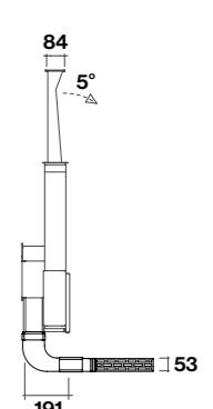
Griglia per aerazione nello zoccolo della cucina, per filtro KACL.951 (opzionale)
