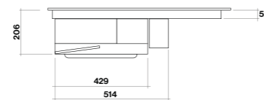
Vista frontale
