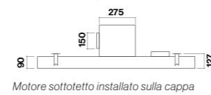
Motore sottotetto installato sulla cappa
