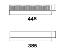
Griglia per aerazione nello zoccolo della cucina, in dotazione con Kit filtro KACL.930
