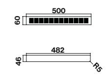
Griglia per aerazione nello zoccolo della cucina, per filtro KACL.951 (opzionale)
