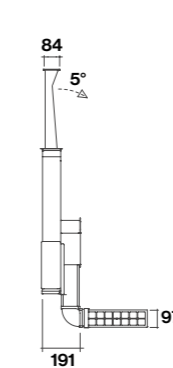
Griglia per aerazione nello zoccolo della cucina, in dotazione con Kit filtro KACL.930
