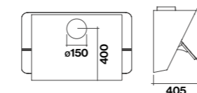
Vista posteriore
