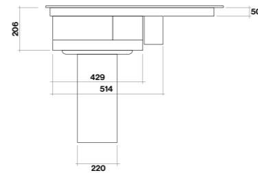
Vista frontale
